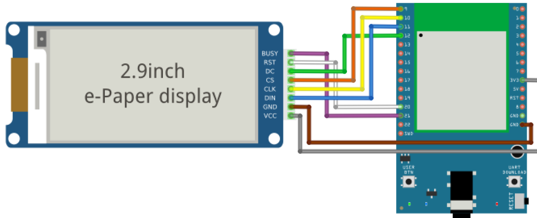
RTL8720DN(BW16) Wiring Diagram:
