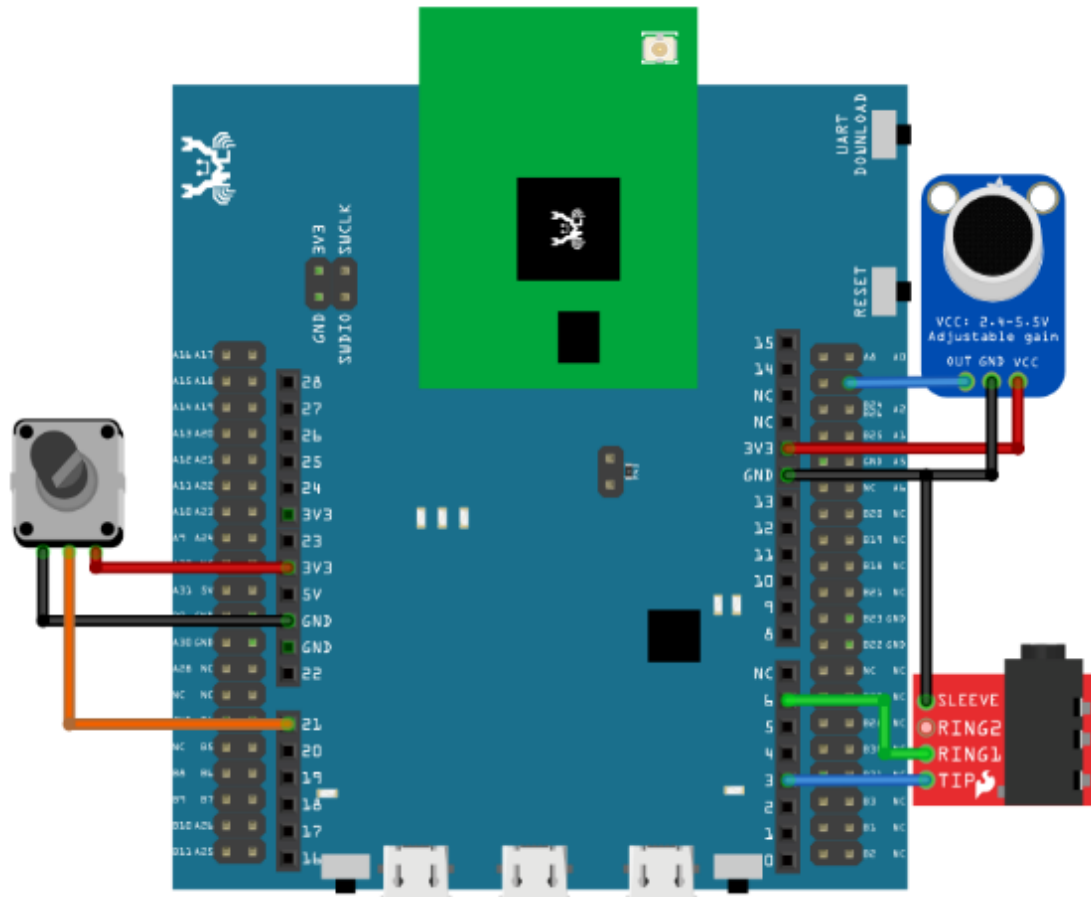
RTL8722DM MINI Wiring Diagram:
