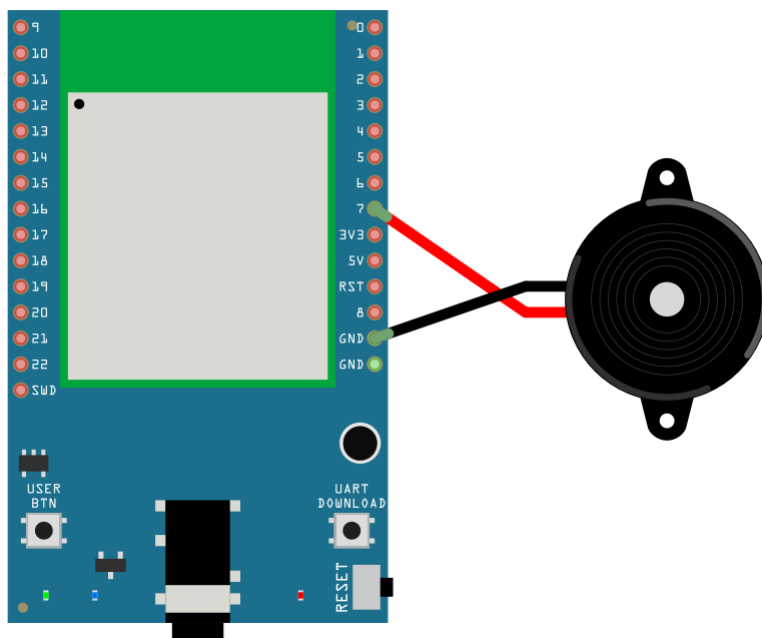
RTL8722DM MINI Wiring Diagram:
