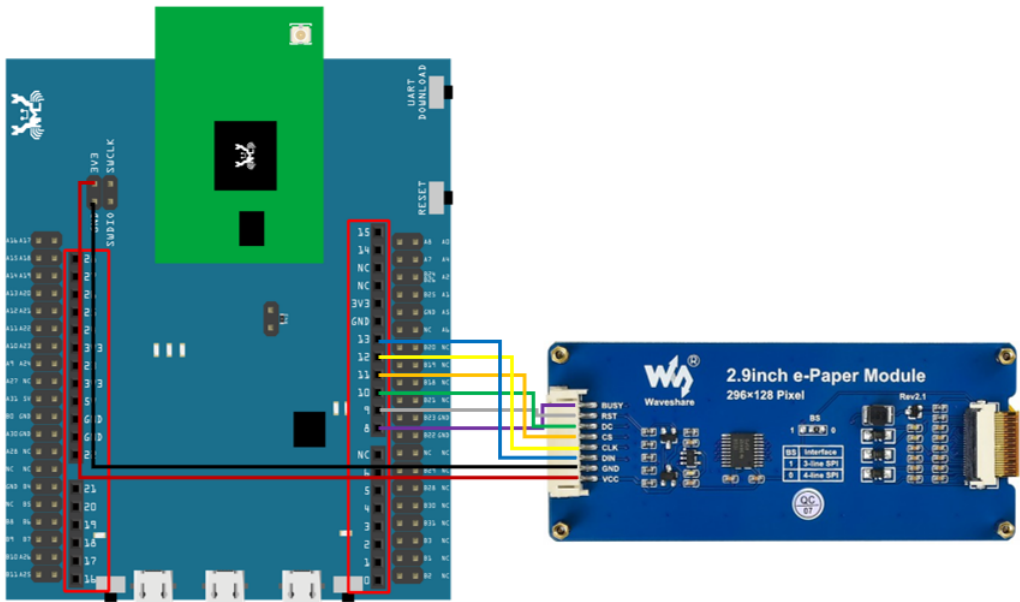
RTL8722DM MINI Wiring Diagram:
