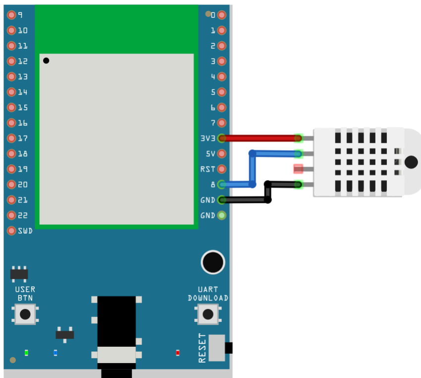
RTL872DM MINI Wiring Diagram:
