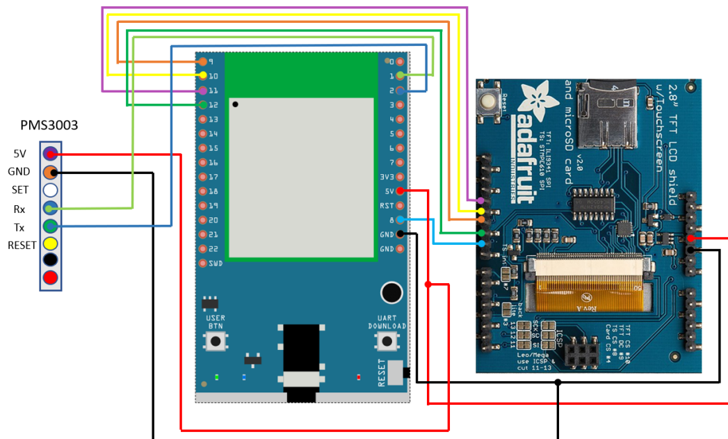
RTL8722DM MINI and and Adafruit 2.8" TFT LCD Wiring Diagram:
