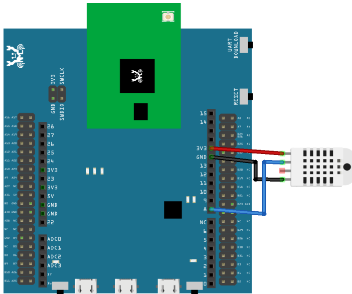
RTL872DM MINI Wiring Diagram:
