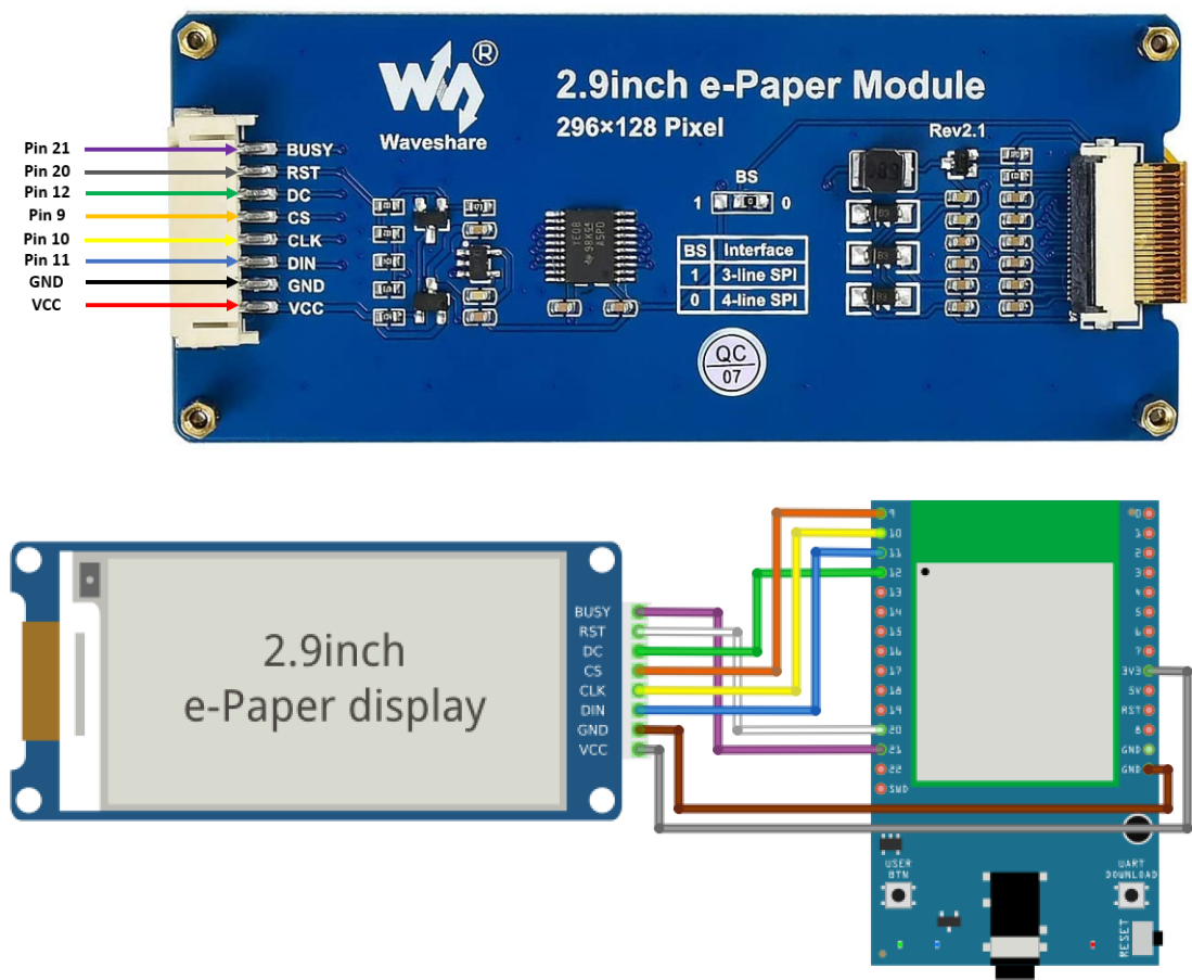
RTL8720DN(BW16) Wiring Diagram:
